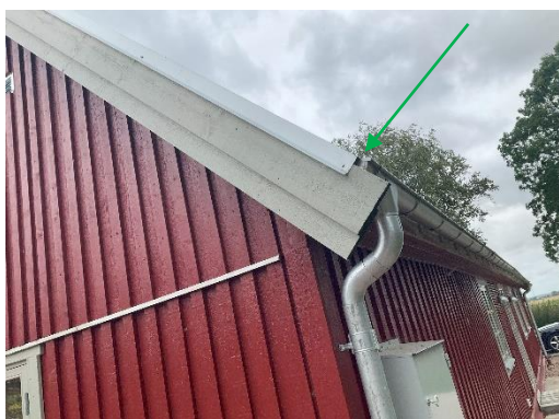
Bild 3: Yttertak. Vindskiveplåt är avslutad i linje med hängrännor
